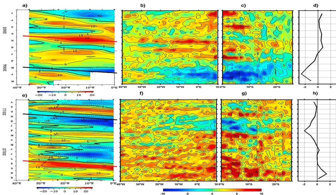
Figure 2 : en haut, de gauche à droite a) diagramme longitude-temps, moyenne sur 5 jours de l'anomalie de la Z20 (m) le long de l'équateur à partir des mesures PIRATA, b) anomalies de la SSH (cm) à partir du produit AVISO le long de l'équateur, c) diagramme longitude-temps des anomalies de SSH (cm) AVISO le long de la côte (0°N-20°S) et d) température associée, de juillet 2003 à mai 2004 ; en bas, e-h) idem d'août 2011 à décembre 2012. D'après Imbol Koungue et al. (2017),
