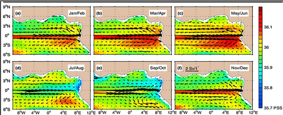
Figure 1 : Climatologie bimensuelle du transport (flèches) et de la salinité (couleurs) au sein de la couche isopycnale 24.5–26.2, déduite du modèle NEMO validé par les mesures in situ (Kolodziejczyk et al., 2014).
